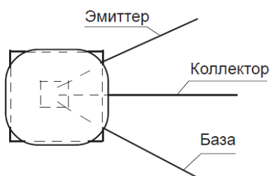
2Т392А-2
